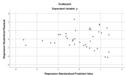
Gambar 2 Uji Heteroskedastitas
