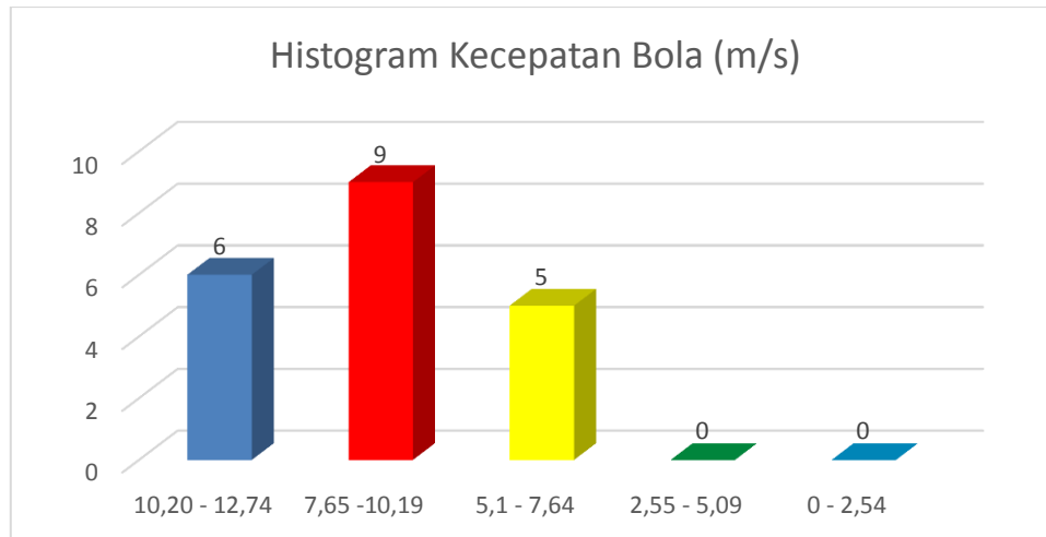
Gambar 2. Histogram Kecepatan Bola (m/s)
