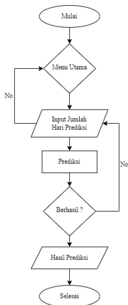
Gambar 1. Flowchart Aplikasi
