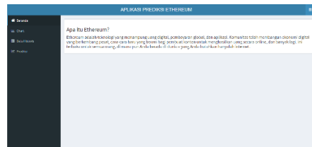
Gambar 6. Halaman Beranda
