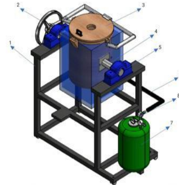
Gambar 2 Alat pelebur limbah kaca dengan kapasitas 5 liter
