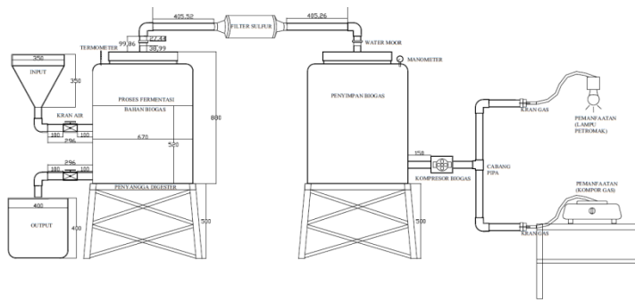
Gambar 3. Rancangan Biodigester
